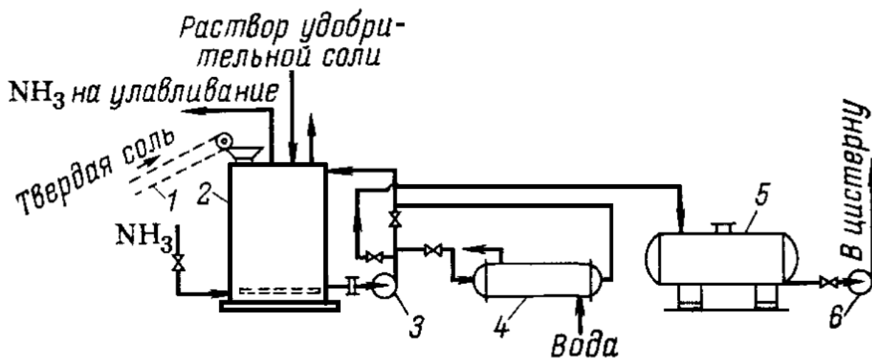
Рис.20 - Схема производства аммиакатов
