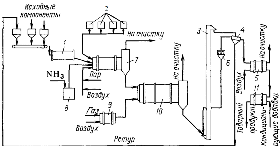
Рисунок 37 - Схема получения сложно-смешанных удобрений:
