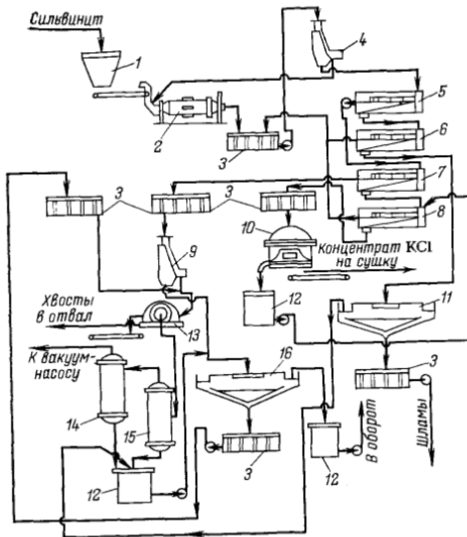
Рисунок 21 - Схема флотационного способа производства хлорида калия с предварительной флотацией глинистого шлама:
