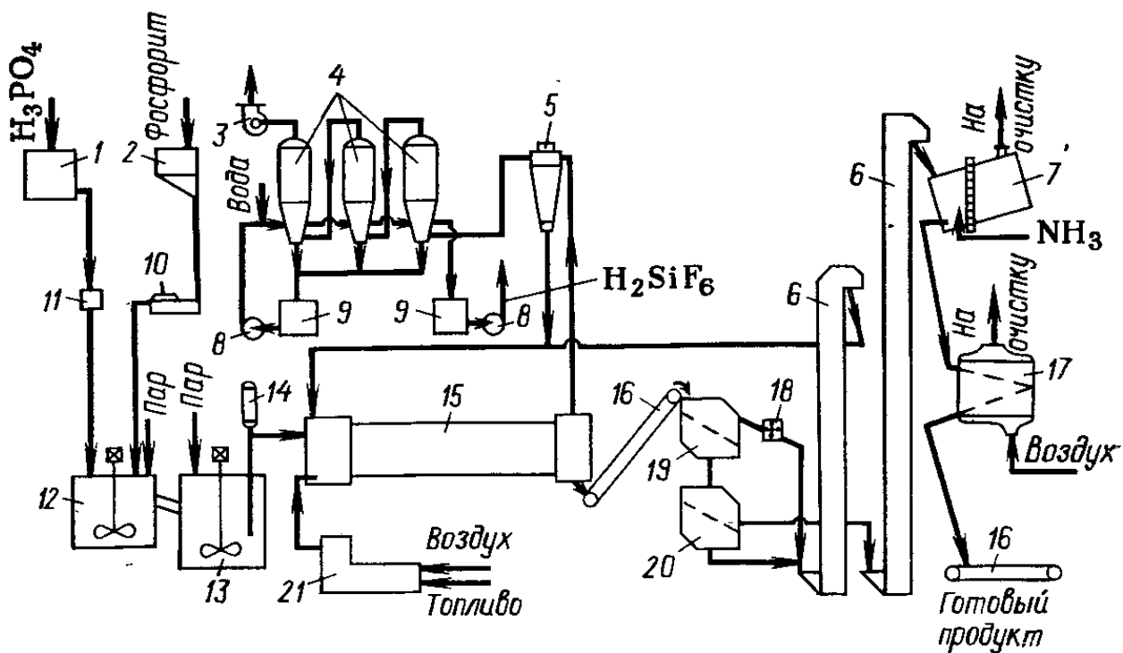
Рисунок 3 - Технологическая схема получения двойного суперфосфата поточным методом:
