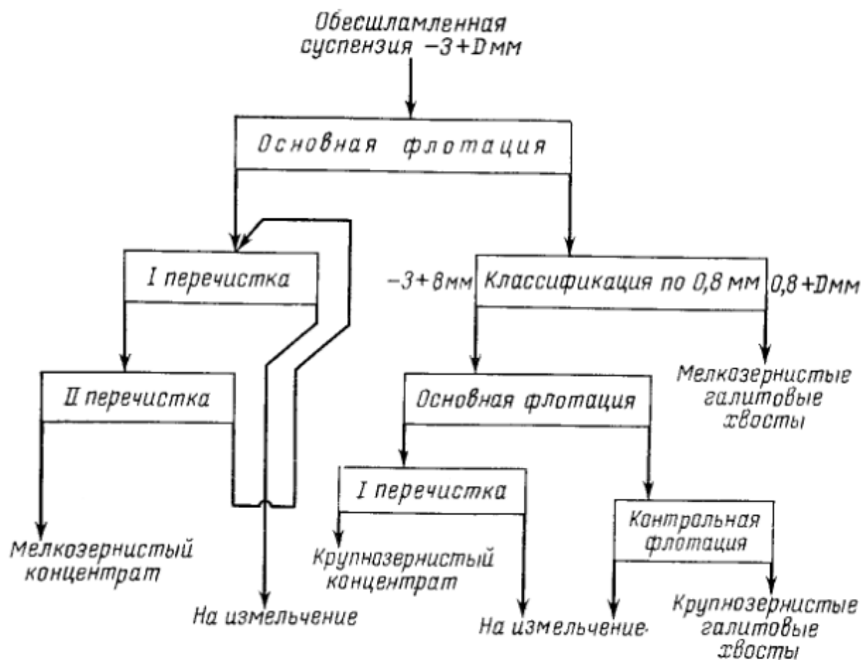
Рисунок 23 - Принципиальная схема циклической флотации сильвинитовых руд для получения крупнозернистого и мелкозернистого концентрата.
