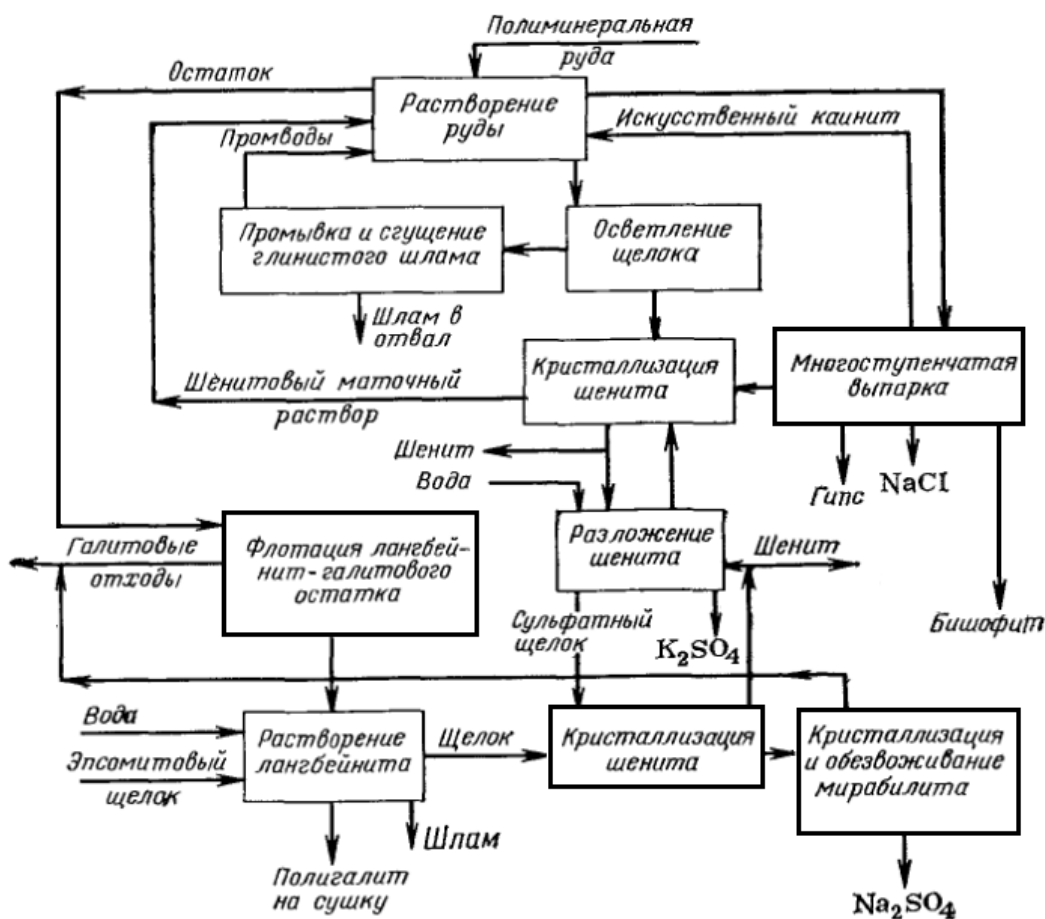
Рис.25 -. Принципиальная схема комплексной переработки полиминеральных руд
