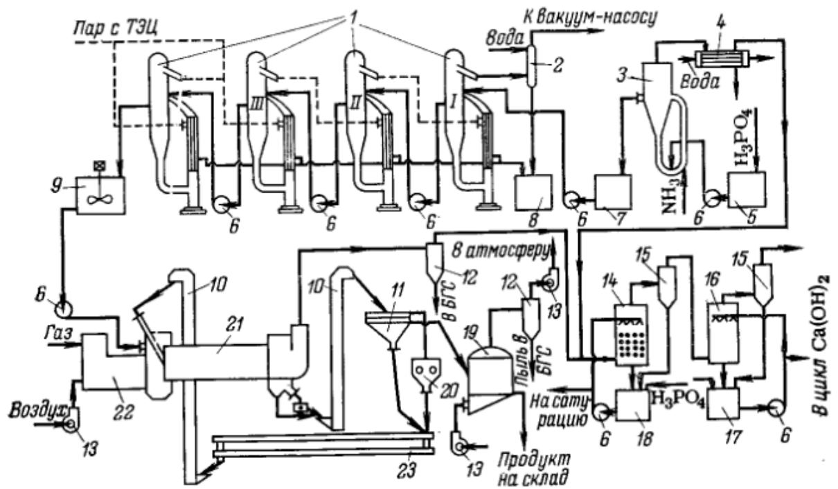
Рисунок 27 - Технологическая схема получения аммофоса с выпариванием пульпы, сушкой и гранулированием в аппарате БГС:
