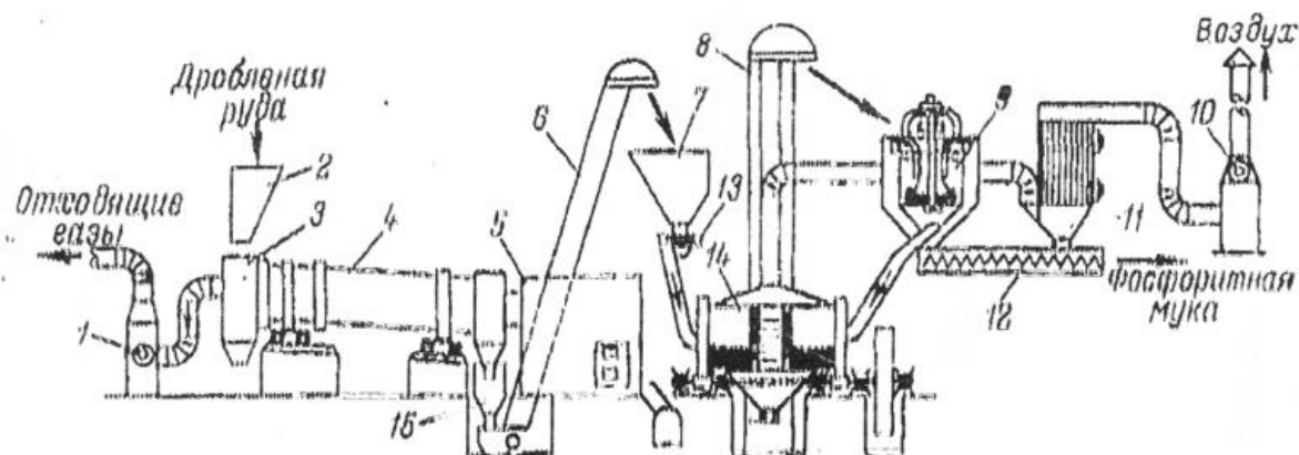
Рисунок 1 - Технологическая схема получения фосфоритной муки:
