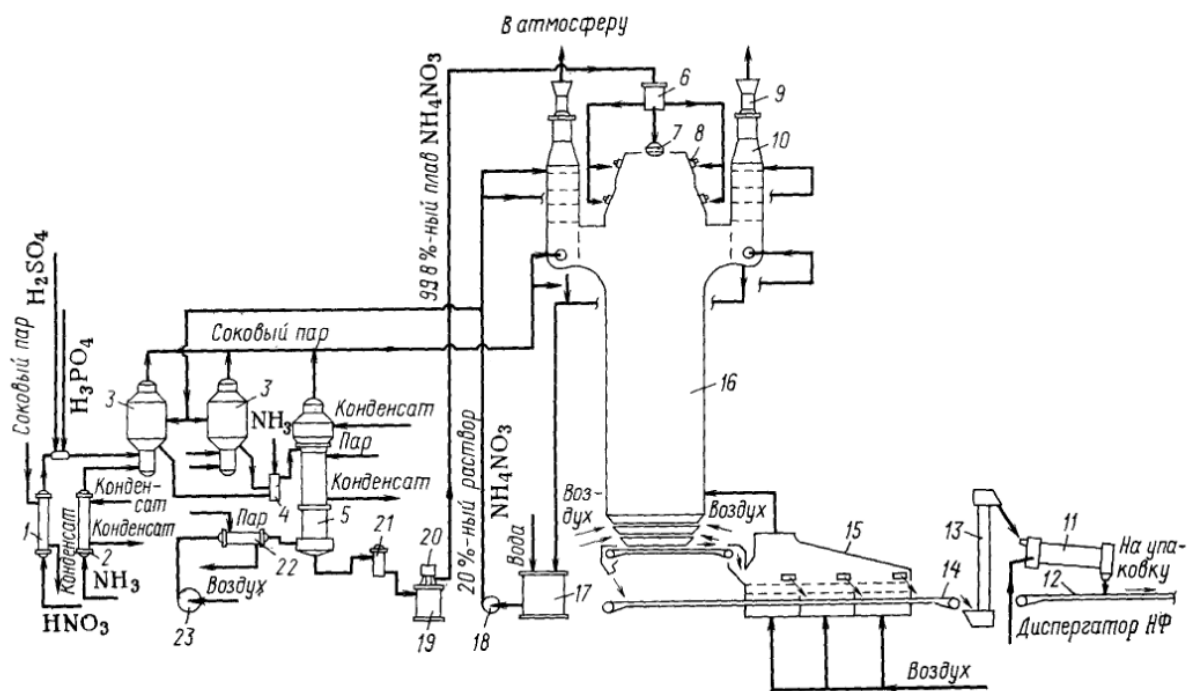
Рис.8. Схема агрегата аммиачной селитры
