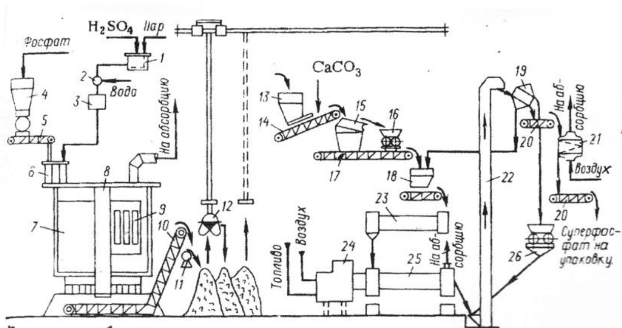
Рисунок 2 - Технологическая схема получения простого гранулированного суперфосфата:
