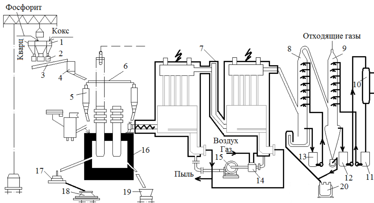
Рисунок 5 - Технологическая схема получения фосфора:
