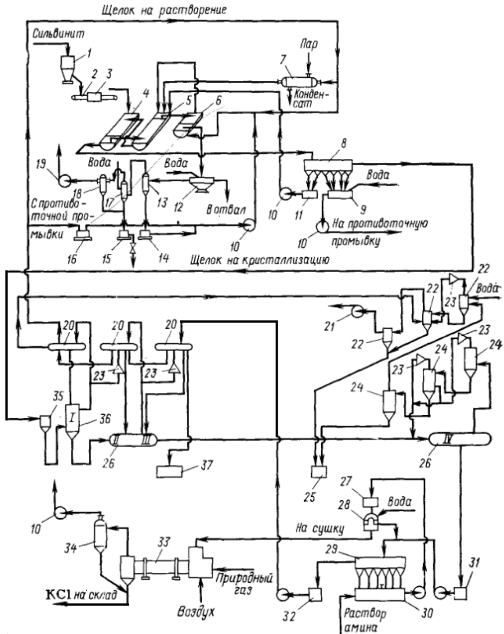
Рис. 24- Схема производства хлорида калия методом растворения и отдельной кристаллизации:
