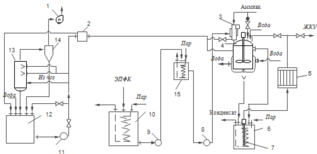
Рисунок 35 - Технологическая схема получения жидких комплексных удобрений:
