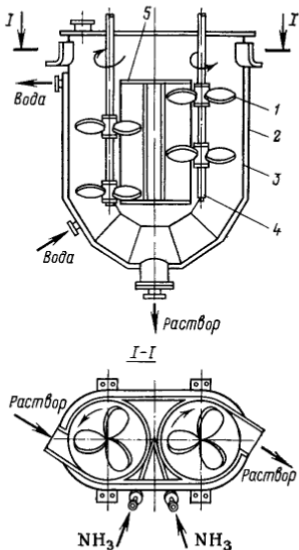
Рисунок 32 - U-образный реактор
