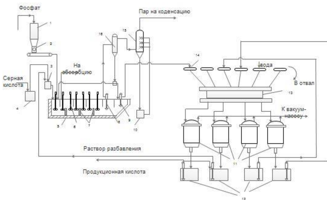
Рисунок 4 - Технологическая схема получения экстракционной фосфорной кислоты: 1-бункер; 2-ленточный дозатор; 3-смеситель; 4,10,12 -сборники; 5-экстрактор; 6- мешалки; 7- перегородка; 8, 9 - погружные насосы; 11 - сепараторы; 13 - подвижная головка вакуум-фильтра; 14 - питающий лоток; 15 - абсорбер фтористых газов; 16 - вакуум-испаритель
