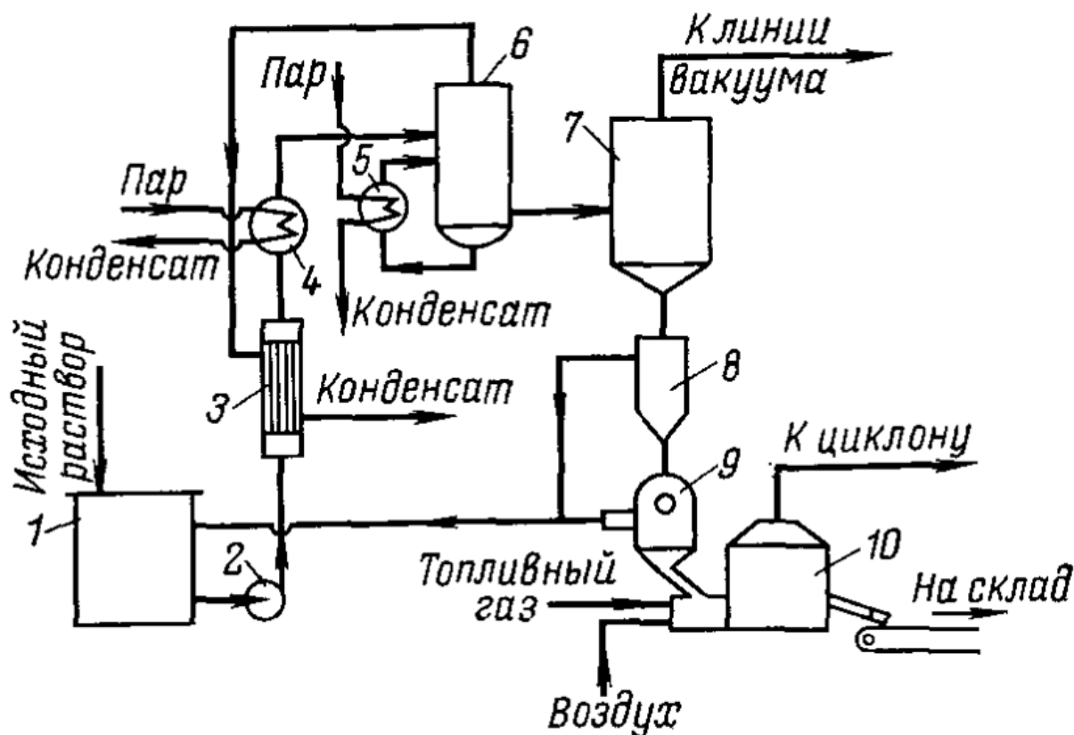
Рис.17. Схема переработки растворов производства капролактама:
