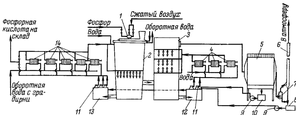
Рис.6. Технологическая схема получения термической фосфорной кислоты:
