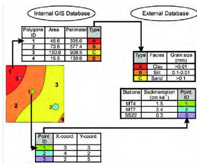
5-сурет. GIS жүйесіндегі төлсипат деректері (Rojas, Vrieling, & Rembold, 2011)
