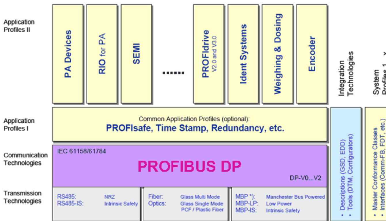
Рис. 3: Структура технической системы PROFIBUS
