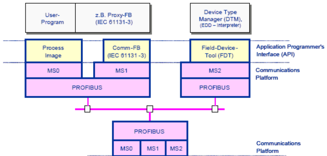
Рис. 28: Интерфейс прикладного программирования, API
