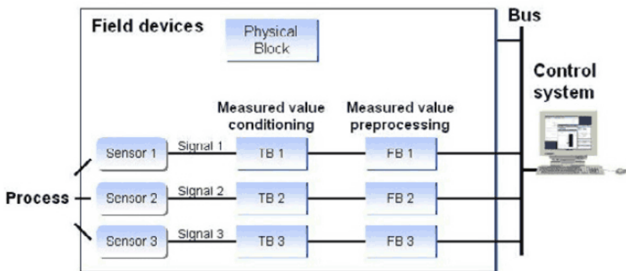
Рис. 22: Блочная структура полевого многофункционального устройства
