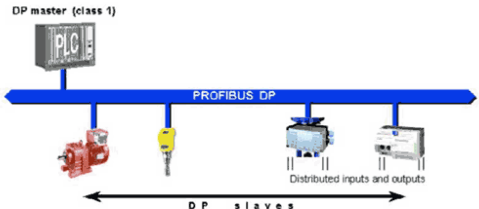
Рис. 10: Система PROFIBUS DP с одним ведущим (mono-master)
