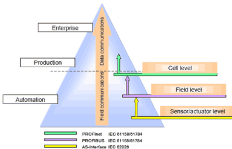
Рис. 1: Коммуникации в технологиях автоматизации
