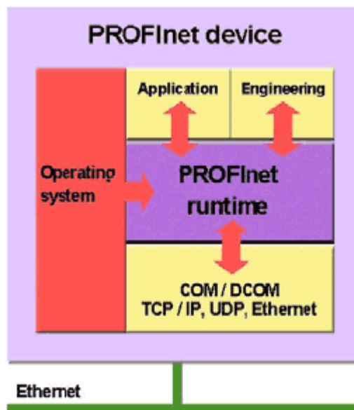
Рис. 35: Структура устройства PROFINet
