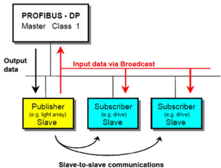
Рис. 15: Обмен данными напрямую между подчиненными устройствами (Slave-to-slave)
