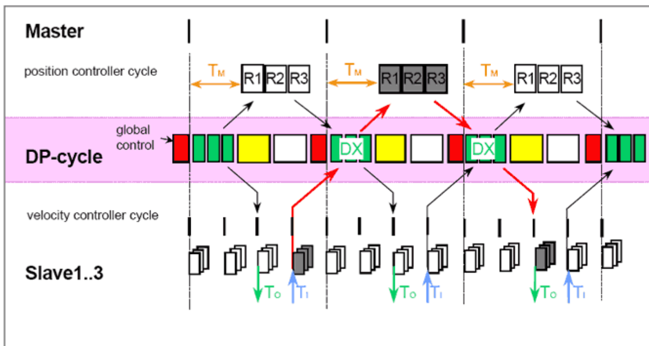
Рис. 14: Изохронный режим
