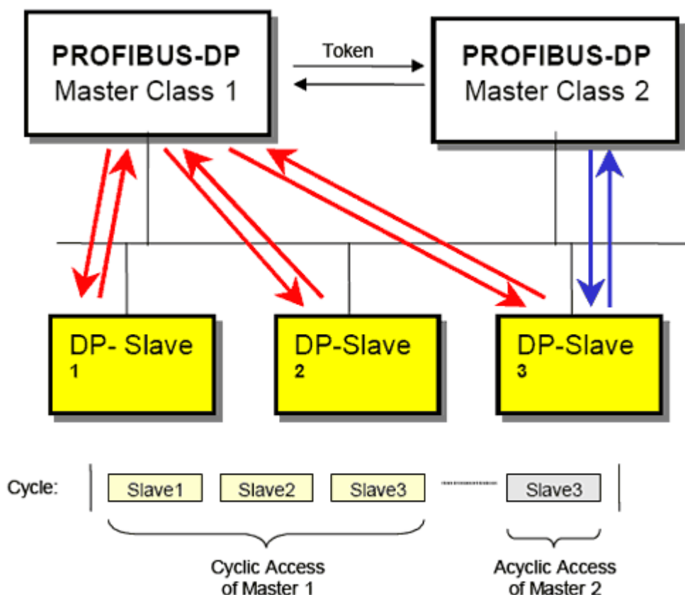
Рис. 13: Циклический и ациклический обмен данными в DP-V1
