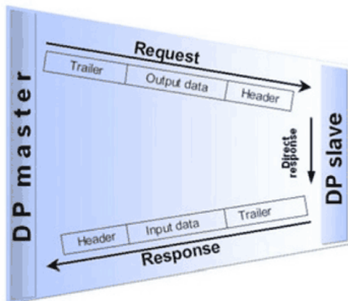
Рис. 11: Циклический обмен пользовательскими данными в DP
