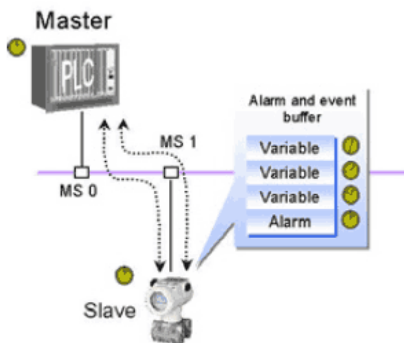
Рис. 19: Отметки времени и сигнальные сообщения
