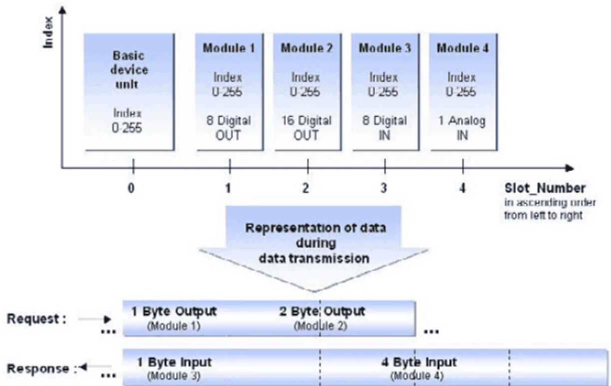
Рис. 16: Адресование с помощью номера слота и индекса
