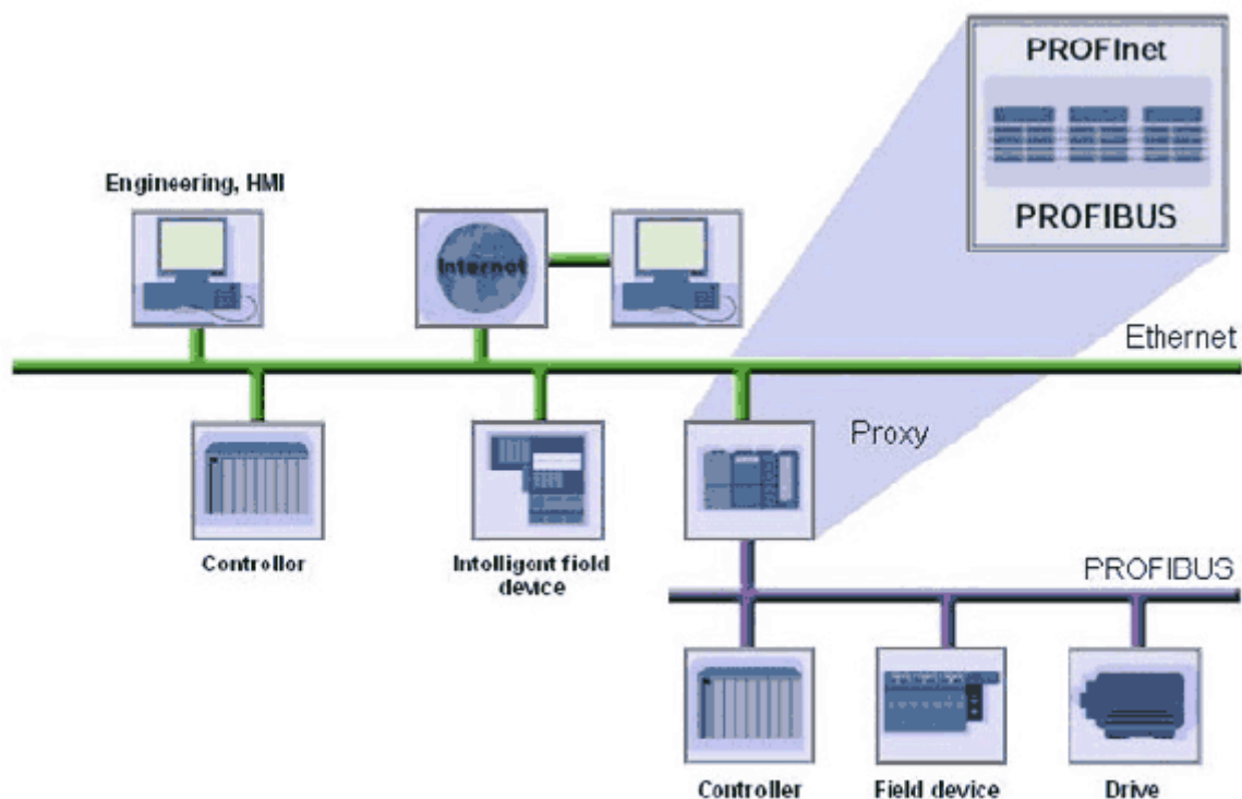
Рис. 36: Модель миграции PROFInet
