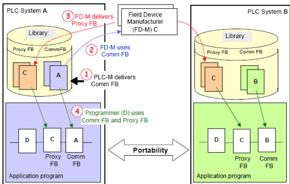
Рис. 29: Портруемый функциональный блок
