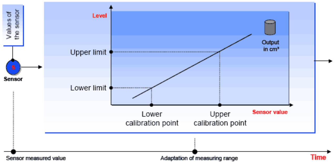
Рис. 23: Спецификация функции калибровки
