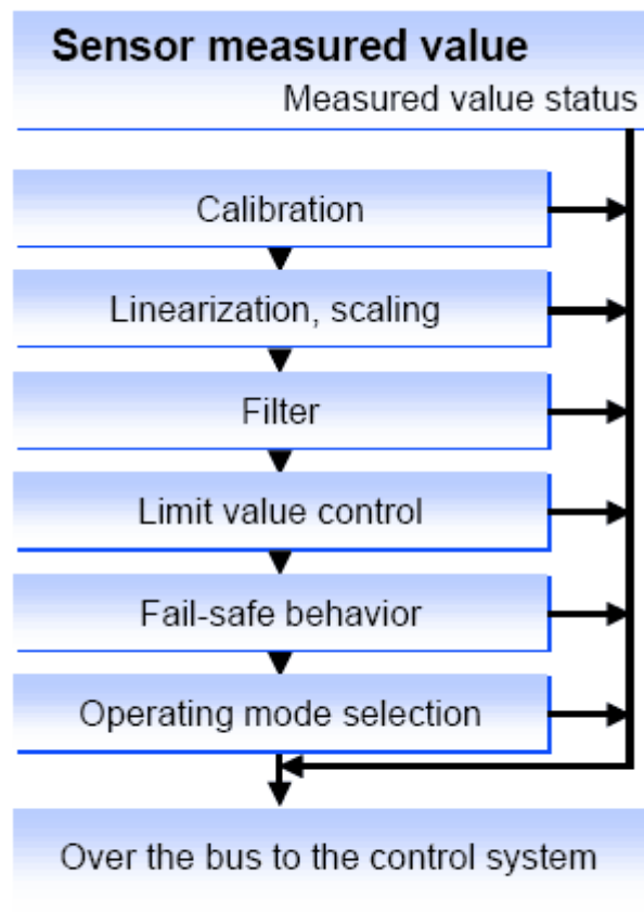
Рис. 25: Цепочка сигналов в профиле PA device
