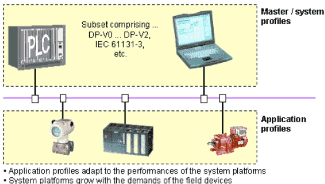
Рис. 27: Системные и прикладные профили (в корреляции)
