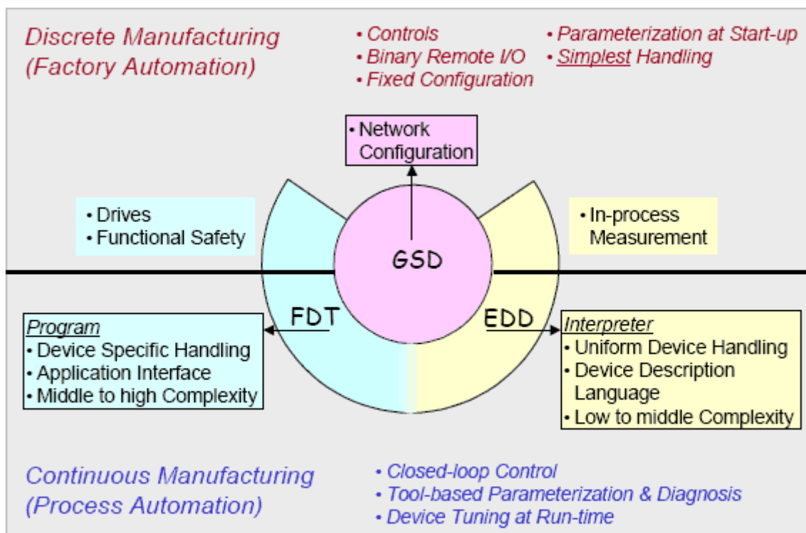
Рис. 30: Технологии интеграции в PROFIBUS
