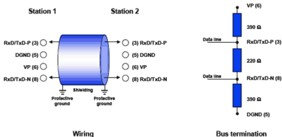
Рис. 6: Прокладка кабеля и шинное окончание в технологии RS485
