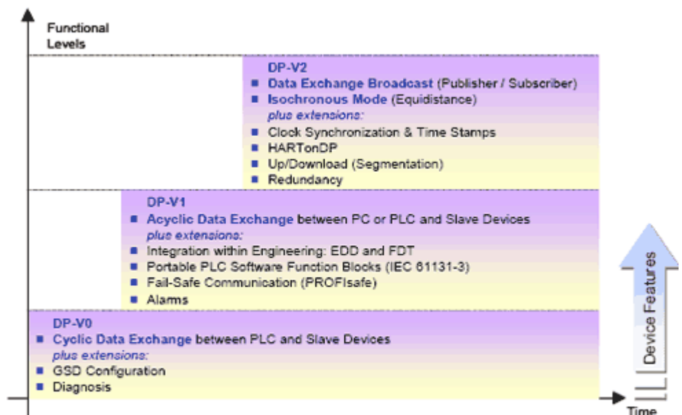
Рис. 8: Ключевые функции версий PROFIBUS DP
