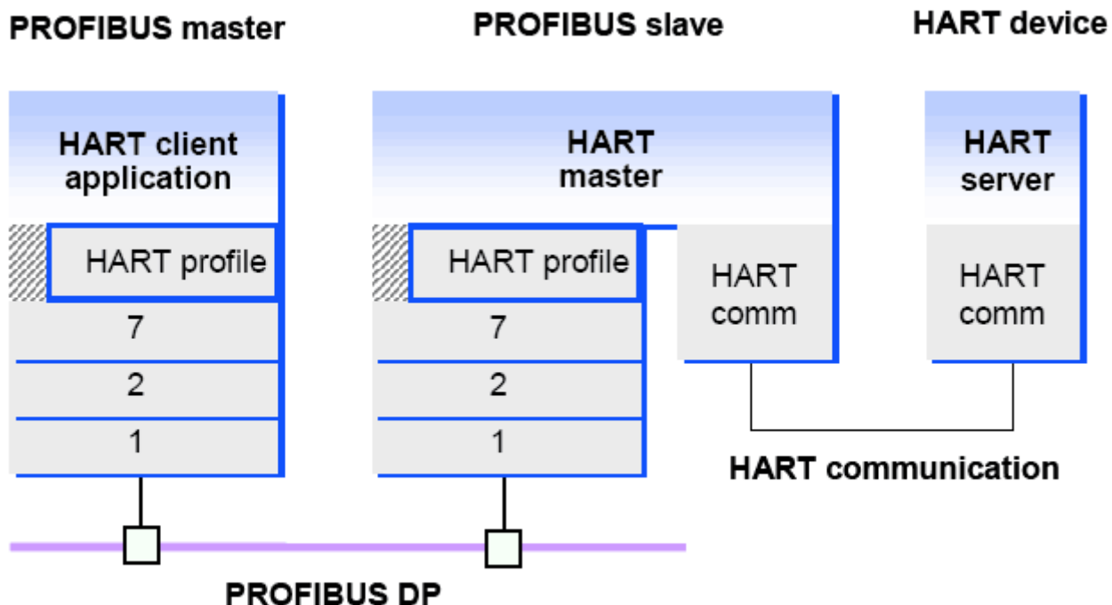
Рис. 18: Интеграция HART устройств в PROFIBUS DP
