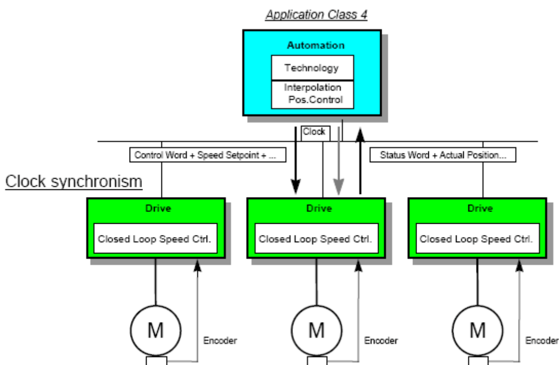
Рис. 21: PROFdrive, позиционирование с интерполяцией и контролем положения
