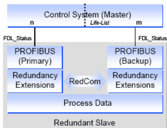
Рис. 20: Резервирование подчиненных устройств
