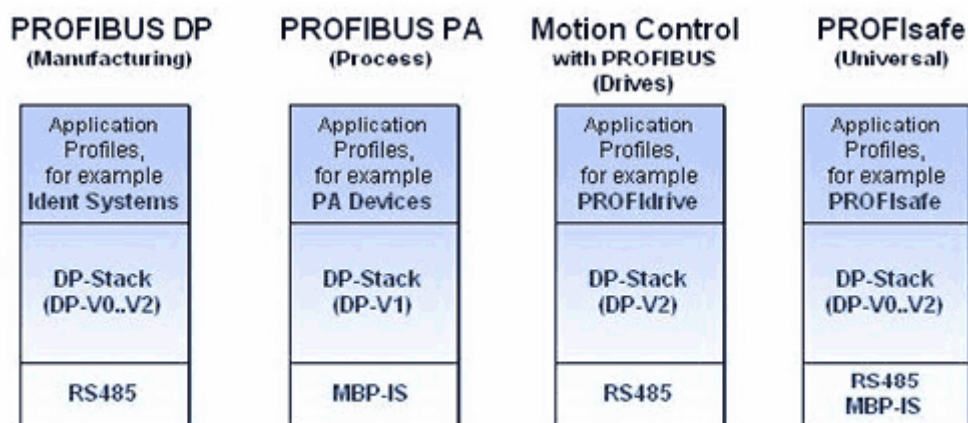
Рис. 4: Типичные прикладные функциональные возможности PROFIBUS
