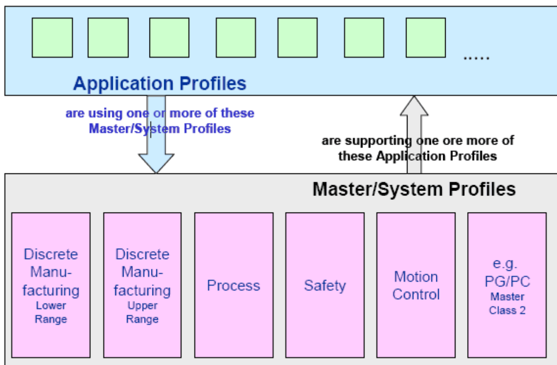
Рис. 26: Ведущие/системные профили для PROFIBUS
