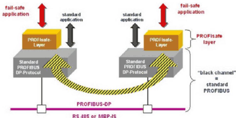
Рис. 17: Безопасный режим с PROFIsafe
