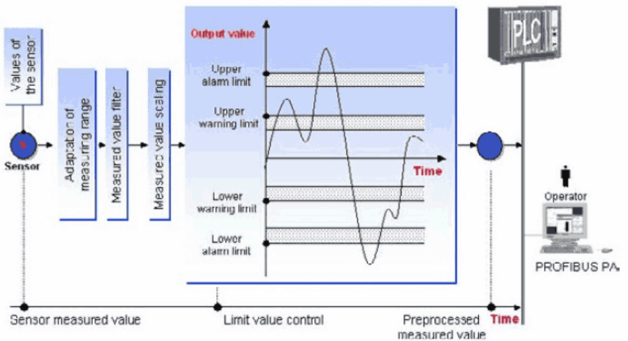
Рис. 24: Спецификация функции проверки предельных значений
