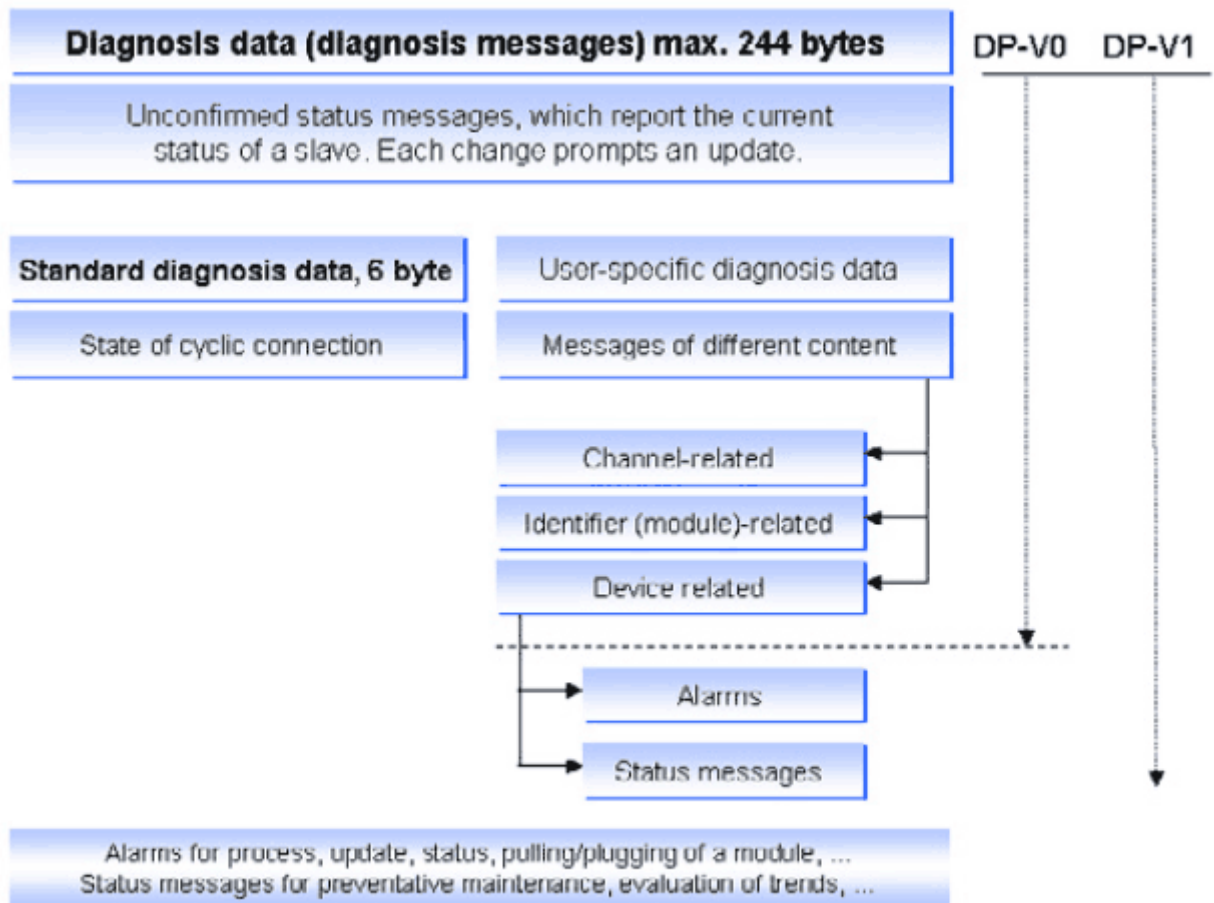
Рис. 12: Конфигурация диагностических сообщений в DP-V0 и DP-V1
