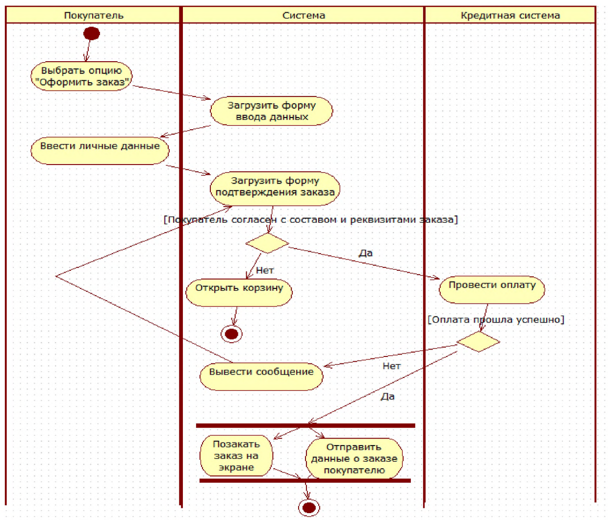
Рисунок 30. Диаграмма деятельности прецедента Оформить заказ
