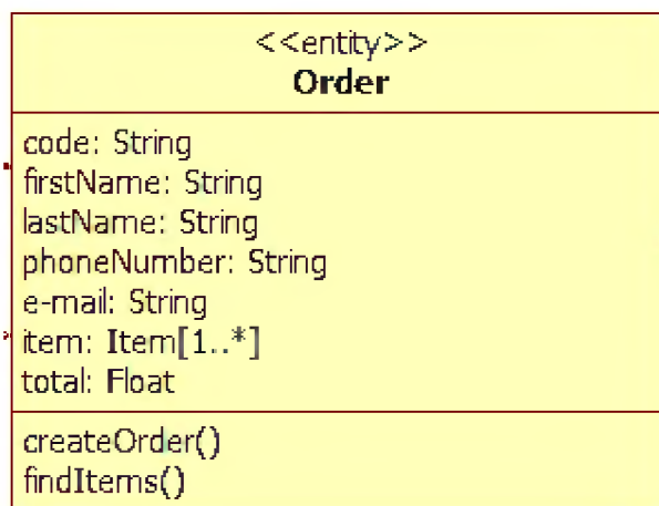
Рисунок 91. Типы атрибутов класса Order
