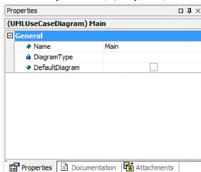
Рисунок 7. Редактор свойств
