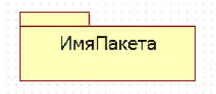
Рисунок 50. Пакет
