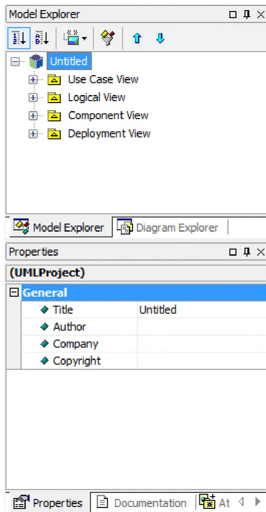
Рисунок 3. Инспектор модели
