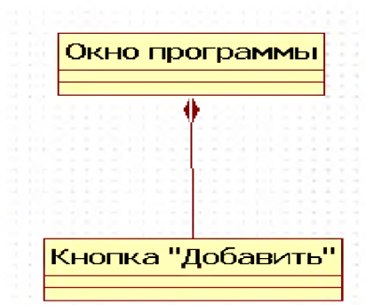
Рисунок 105. Композиция
