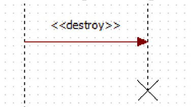
Рисунок 63. Уничтожение объекта
