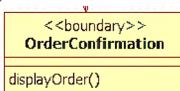
Рисунок 77. Операция класса
