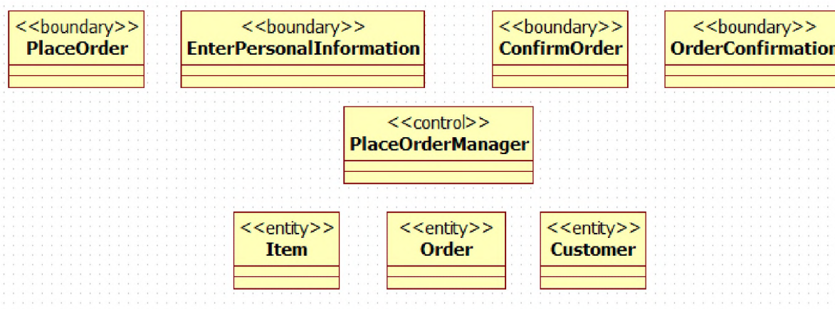
Рисунок 46. Диаграмма классов сценария Оформление заказа со стереотипами
