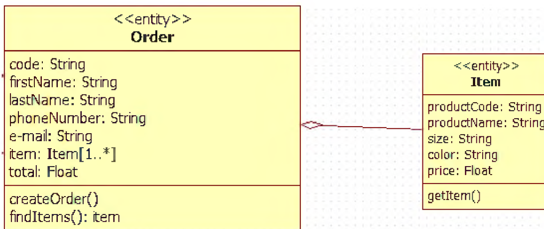
Рисунок 104. Агрегация между классами Товар и Заказ
