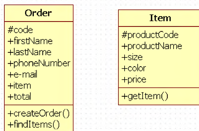
Рисунок 86. Атрибуты классов Товар и Заказ с видимостью
