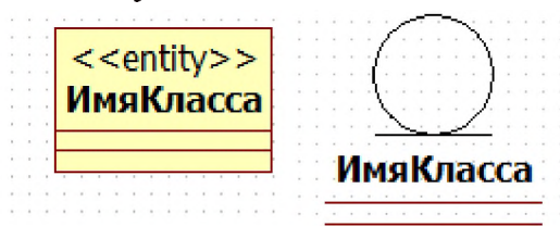
Рисунок 35. Обозначение классов-сущностей
