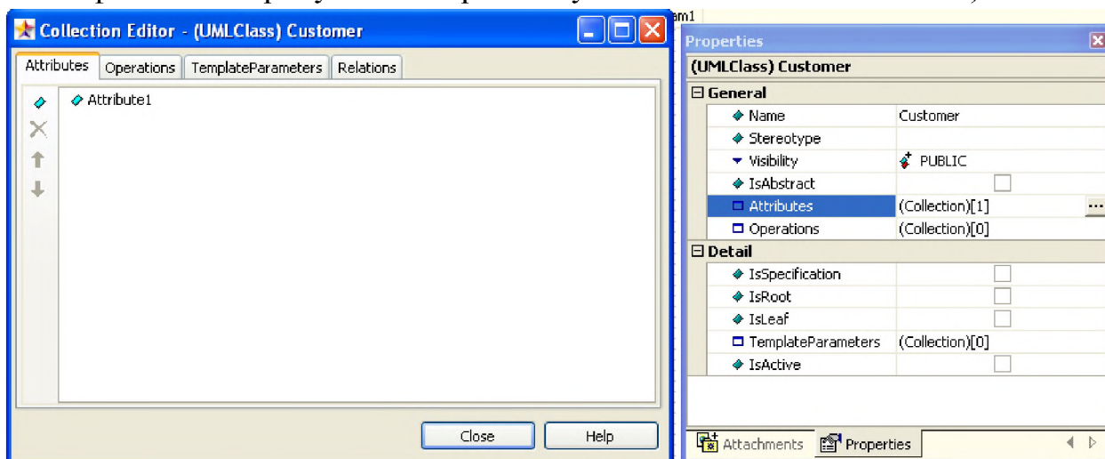
Рисунок 75. Создание атрибута
