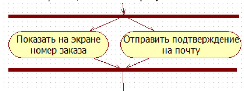
Рисунок 27. Линии синхронизации
