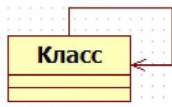
Рисунок 99. Рефлексивная ассоциация
