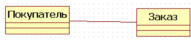
Рисунок 97. Двунаправленная ассоциация
