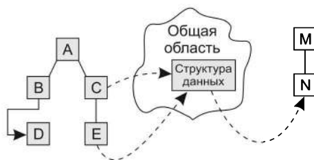
Рис. 6.20. Сцепление по общей области и содержанию
