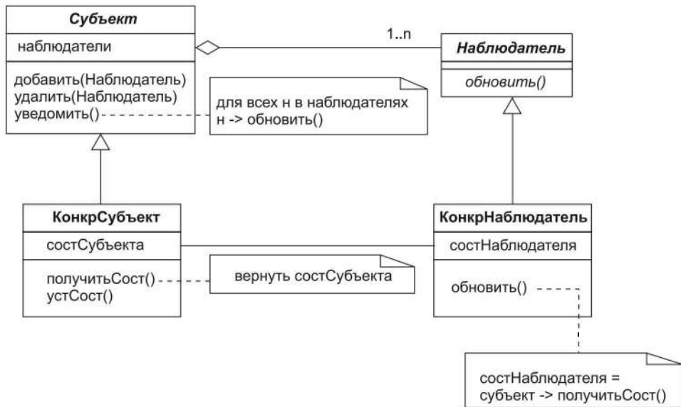
Рис. 10.47. Структурная составляющая паттерна Наблюдатель
