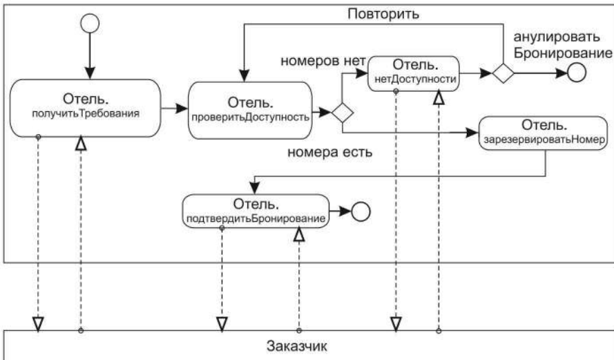
Рис. 18.10. Фрагмент рабочего потока бронирования номеров
