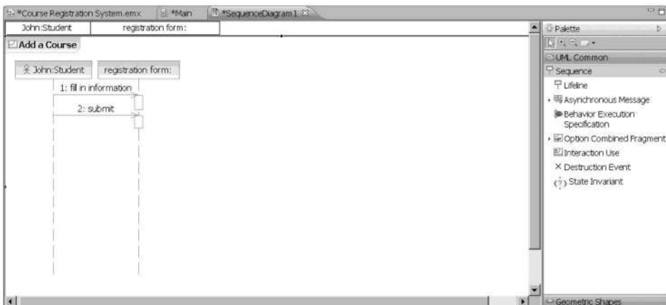
Рис. 21.25. Диаграмма последовательности после добавления registration form
