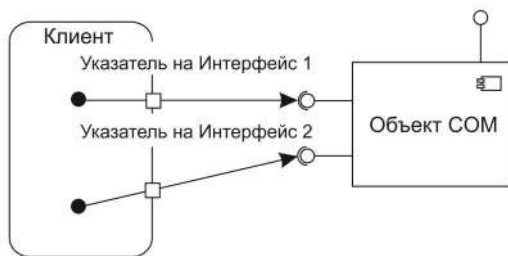
Рис. 10.62. Доступ клиента к интерфейсам объекта COM
