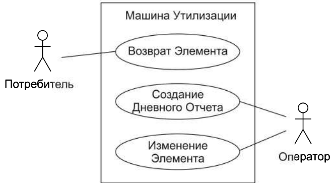
Рис. 9.12. Диаграмма Use Case для машины утилизации
