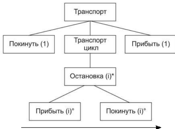
Рис. 5.14. Объектная структура для транспорта
