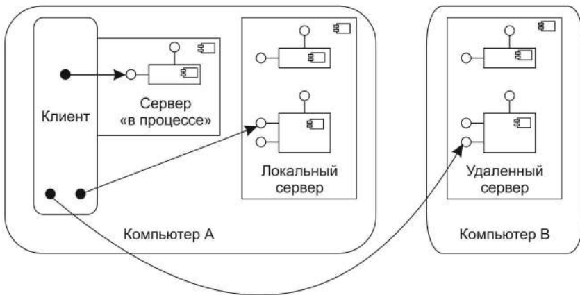
Рис. 10.65. Различные серверы COM-объектов
