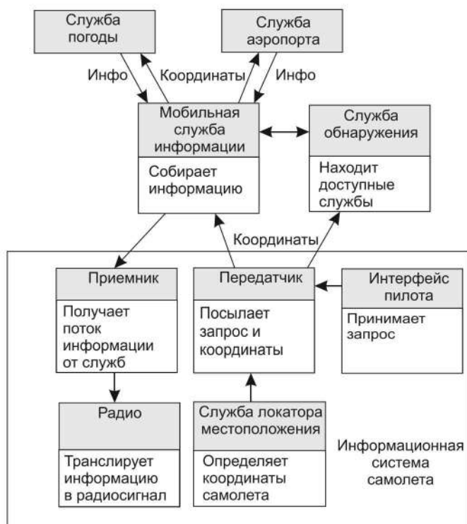
Рис. 18.5. Сервисно-ориентированная информационная система самолета
