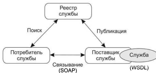
Рис. 18.3. Замысел сервисно-ориентированной архитектуры
