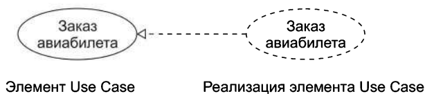
Рис. 10.42. Элемент Use Case и его реализация
