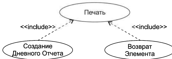
Рис. 9.15. Применение отношения включения
