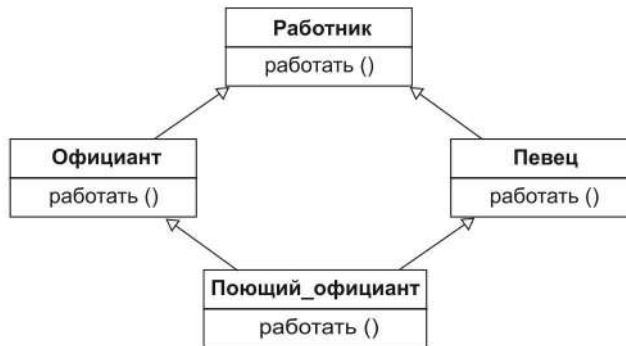
Рис. 10.29. Ромбовидная решетка наследования
