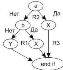
Рис. 14.5. Преобразованный потоковый граф
