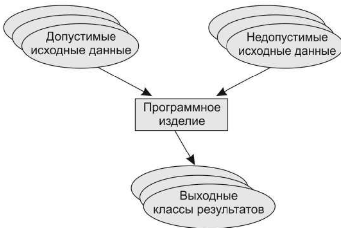
Рис. 15.2. Разбиение по эквивалентности
