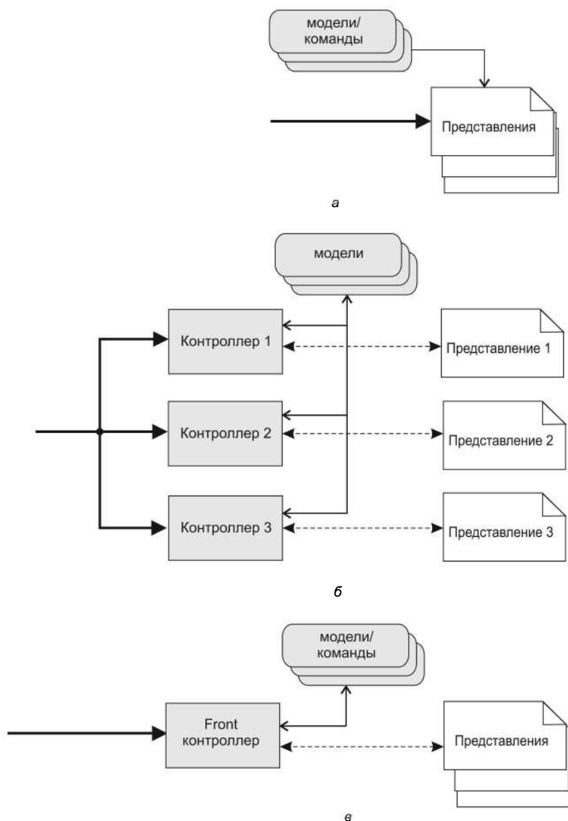
Рис. 19.8. Структура сервера приложения: а — на основе Template View; б — на основе Page Controller; в — на основе Front Controller
