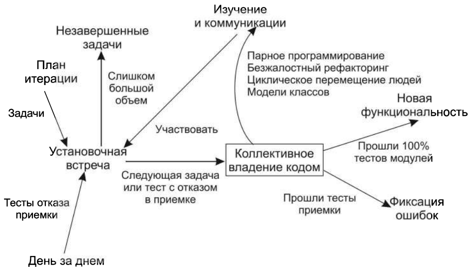
Рис. 13.33. Структура элемента XP-разработки
