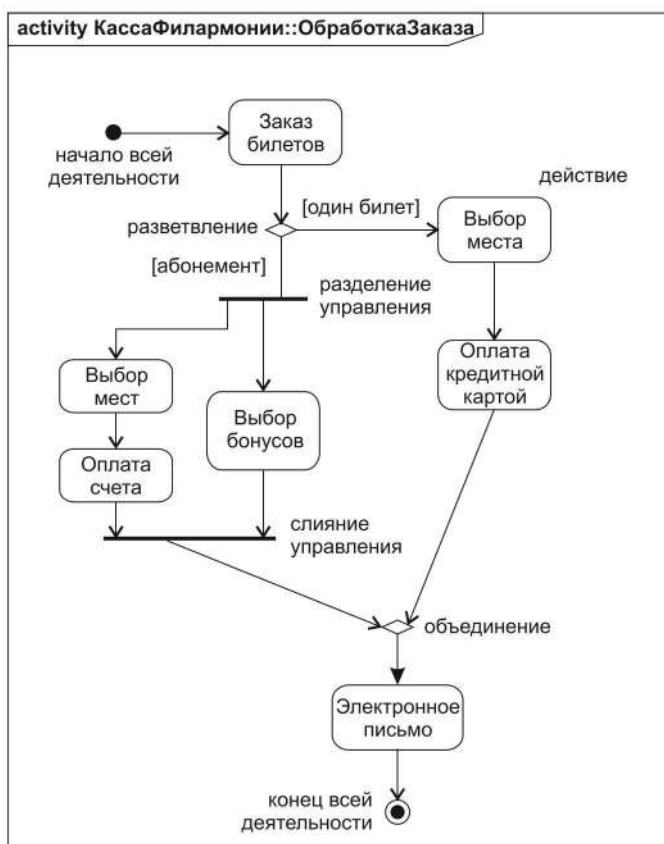
Рис. 9.19. Диаграмма деятельности для покупки билета в филармонию
