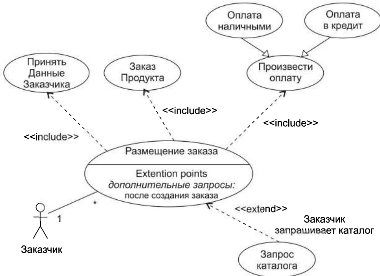
Рис. 9.9. Диаграмма Use Case для обслуживания заказчика
