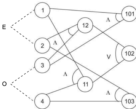
Рис. 15.14. Граф причинно-следственных связей
