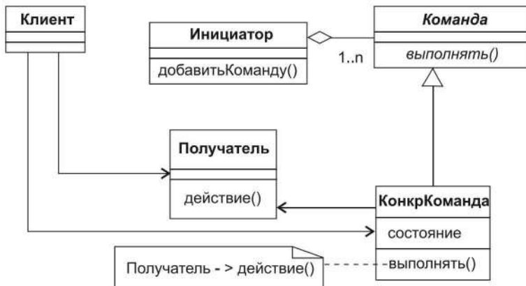
Рис. 10.54. Структурная составляющая паттерна Команда
