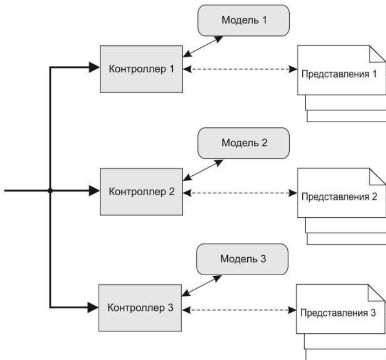
Рис. 19.7. Обобщенная структура категории Модель-Представление-Контроллер
