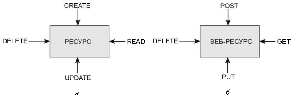
Рис. 18.6. Операции над ресурсами: а — обычные; б — методы HTTP
