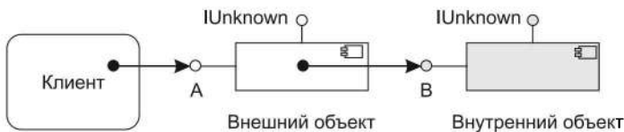
Рис. 10.68. Повторное использование COM-объекта с помощью включения
