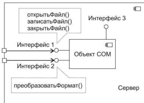
Рис. 10.61. Организация объекта COM
