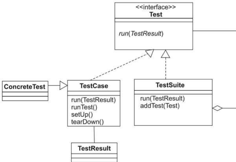
Рис. 17.4. Базовая структура среды JUnit
