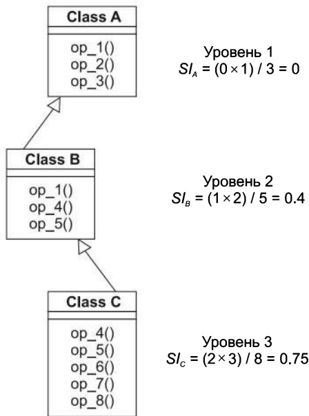
Рис. 12.8. Расчет индексов специализации классов
