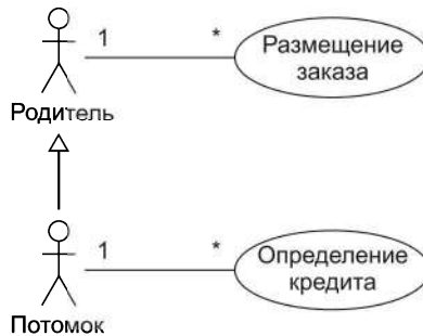
Рис. 9.4. Отношение обобщения между актерами
