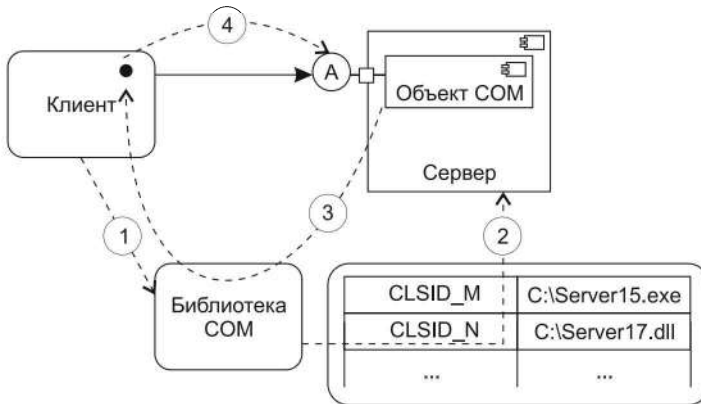
Рис. 10.66. Создание одиночного COM-объекта. Клиент вызывает coCreateInstance (CLSID M, IID A) (1); библиотека COM находит сервер и запускает его (2); библиотека COM возвращает указатель на интерфейс A (3); теперь клиент может вызывать операции COM-объекта (4)
