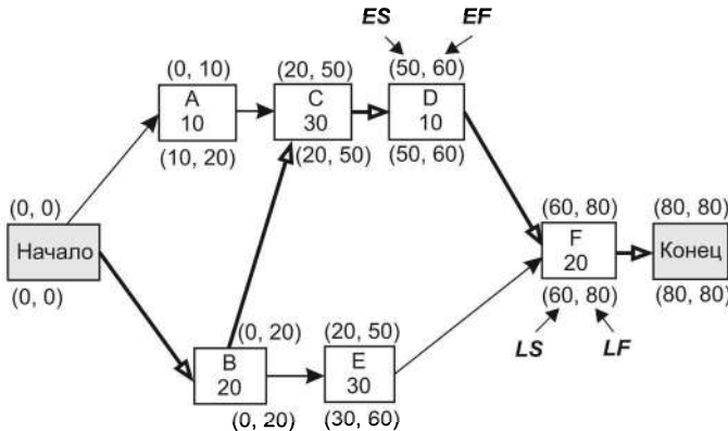
Рис. 2.6. Пример диаграммы предшествования
