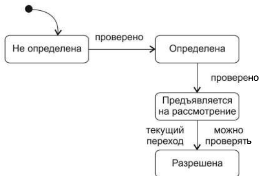
Рис. 17.3. Тестирование «преимущественно в ширину»
