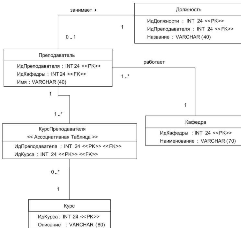
Рис. 11.23. Отношения между таблицами реляционной БД
