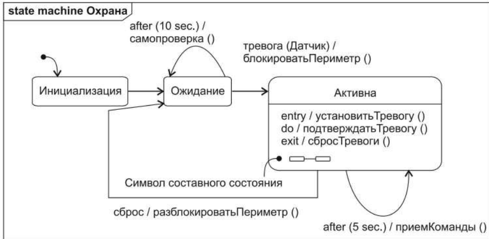
Рис. 9.37. Диаграмма конечного автомата для системы охранной сигнализации
