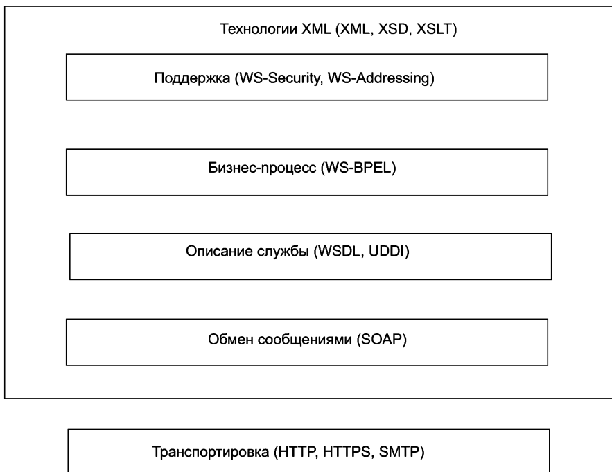
Рис. 18.4. Стек протоколов для веб-служб
