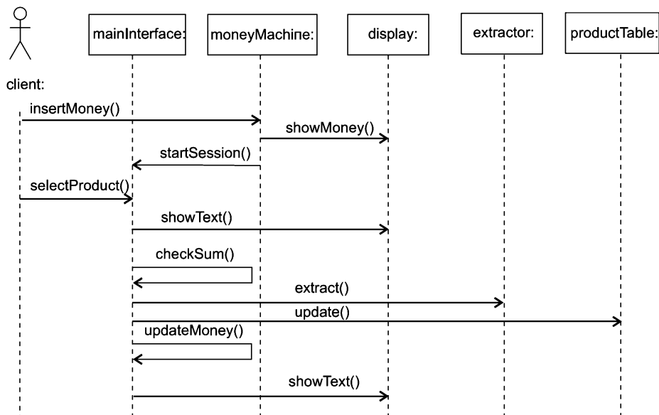
Рис. 13.22. Диаграмма последовательности для элемента Use Case Buy
