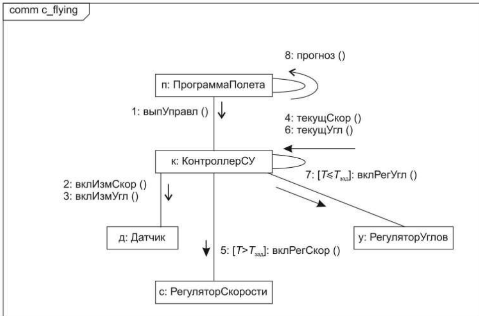
Рис. 9.26. Диаграмма коммуникации системы управления полетом
