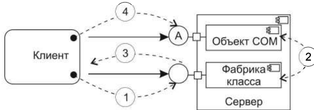
Рис. 10.67. Создание COM-объекта с помощью фабрики класса. Клиент вызывает IClassFactory::createInstance (IID A) (1) ; фабрика класса создает COM-объект и получает указатель на его интерфейс (2); фабрика класса возвращает указатель на интерфейс A COM-объекта (3); теперь клиент может вызывать операции COM-объекта (4)
