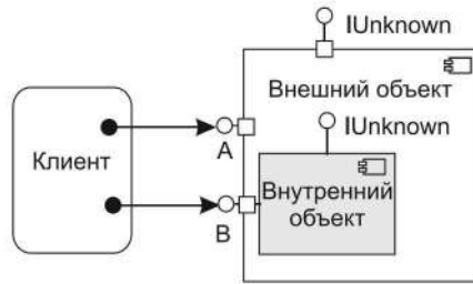
Рис. 10.69. Повторное использование COM-объекта с помощью агрегирования
