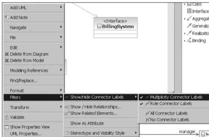
Рис. 21.39. Выбор степени подробности информации об отношении
