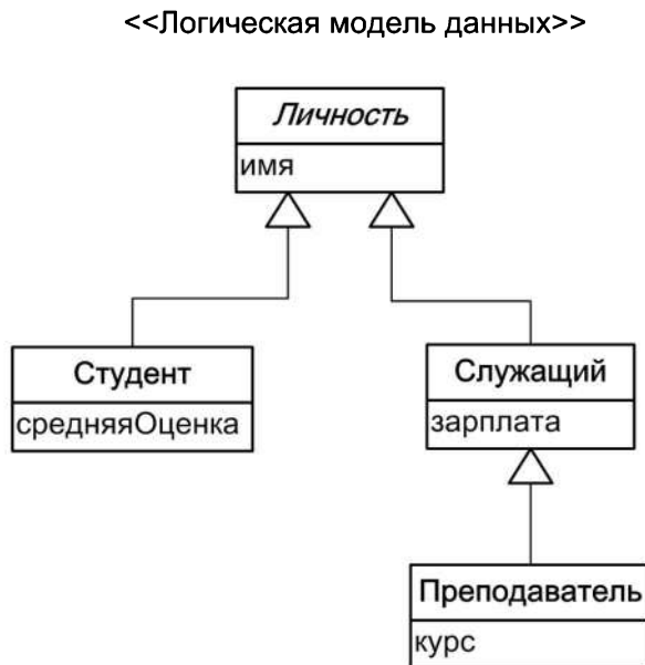
Рис. 11.12. Отображаемое дерево наследования классов
