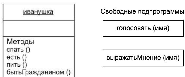
Рис. 8.2. Методы и свободные подпрограммы
