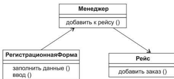
Рис. 10.44. Статическая составляющая кооперации Заказ авиабилета
