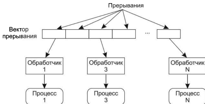
Рис. 6.14. Система, управляемая прерываниями
