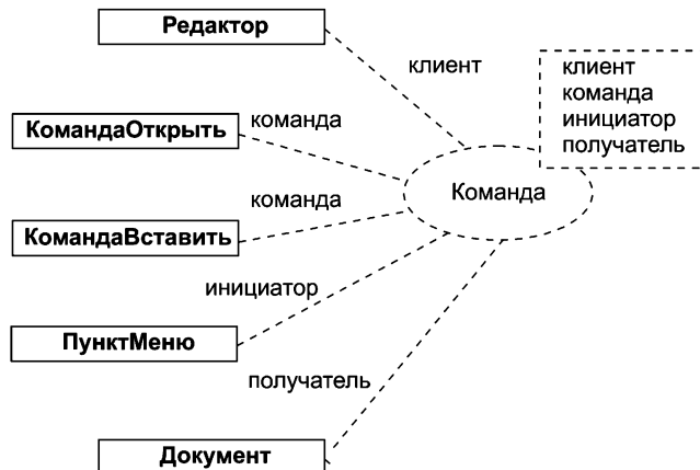
Рис. 10.56. Настройка паттерна Команда
