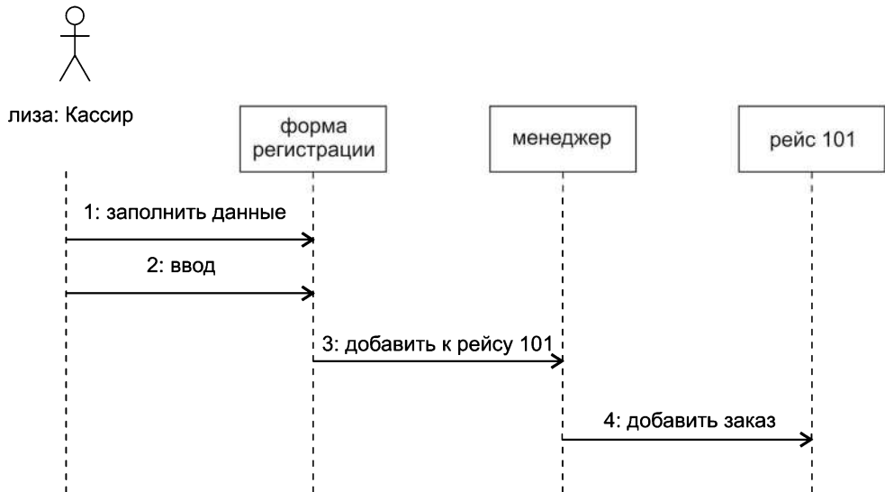
Рис. 10.43. Динамическая составляющая кооперации Заказ авиабилета
