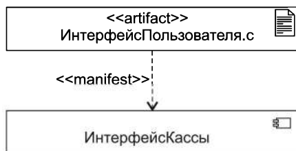
Рис. 10.72. Пример артефакта и реализуемого им компонента
