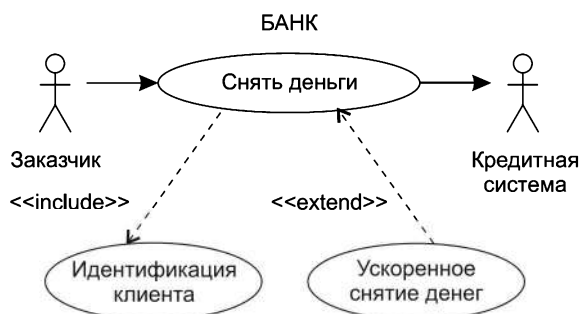
Рис. 9.8. Простейшая диаграмма Use Case для банка
