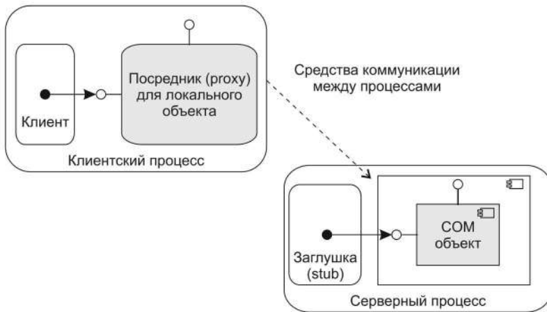
Рис. 10.70. Организация маршалинга и демаршалинга
