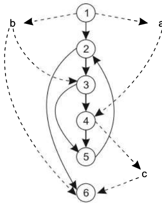
Рис. 14.10. Граф программы с управляющими и информационными связями
