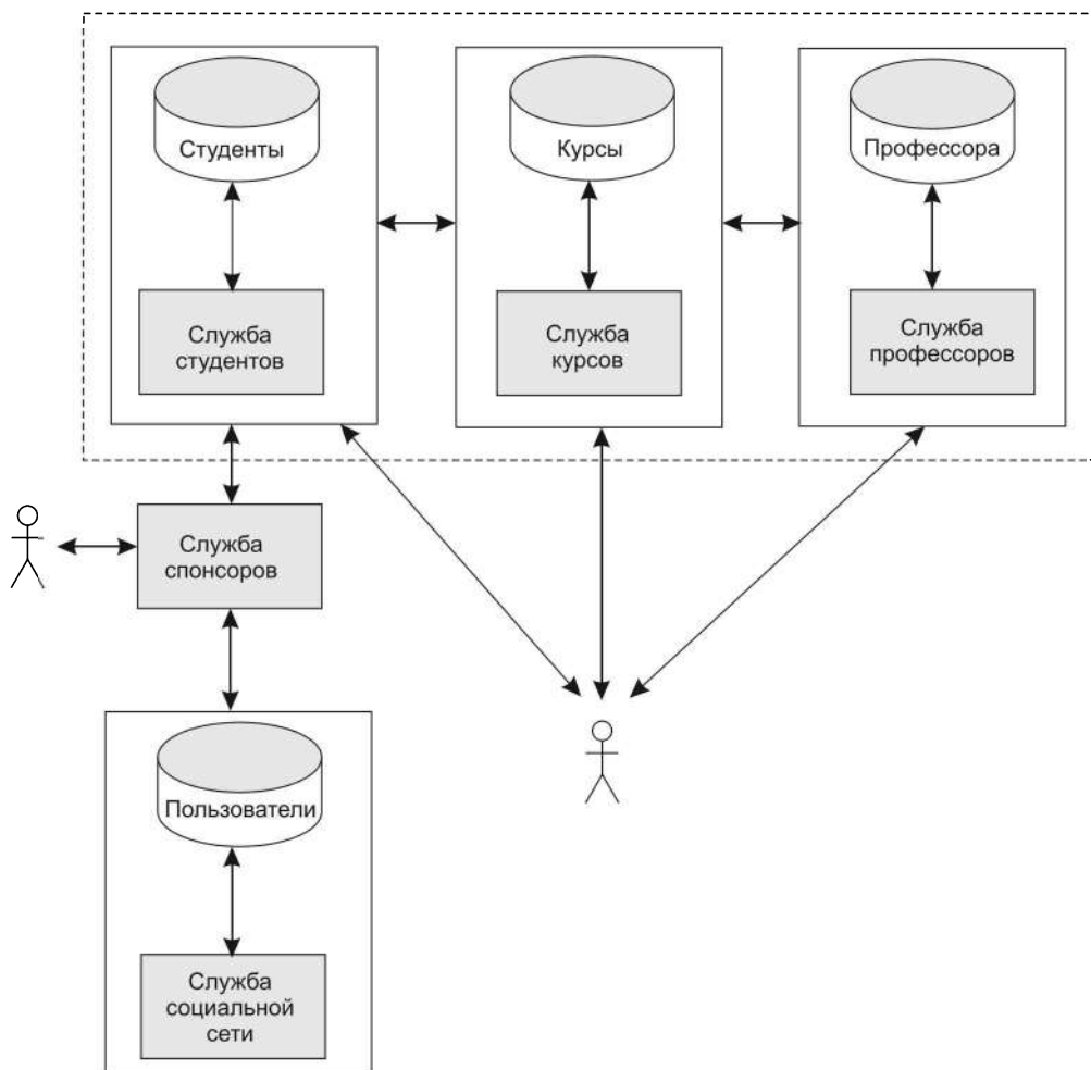
Рис. 18.2. Сервисно-ориентированная информационная система университета
