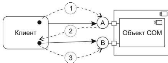
Рис. 10.64. Получение указателя на интерфейс с помощью queryInterface .
