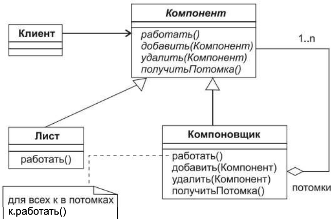
Рис. 10.51. Структурная составляющая паттерна Компоновщик
