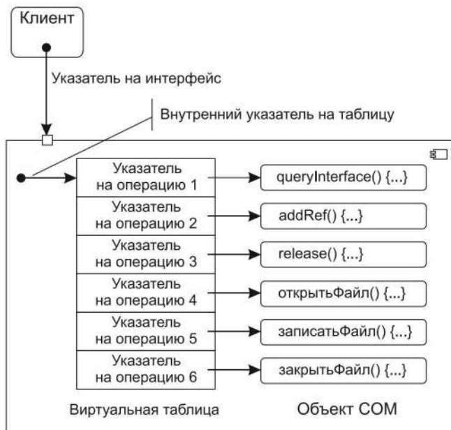
Рис. 10.63. Внутренняя структура интерфейса IRabotaCFайлами
