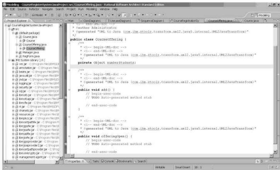
Рис. 21.55. Сгенерированный код Java для класса CourseOffering
