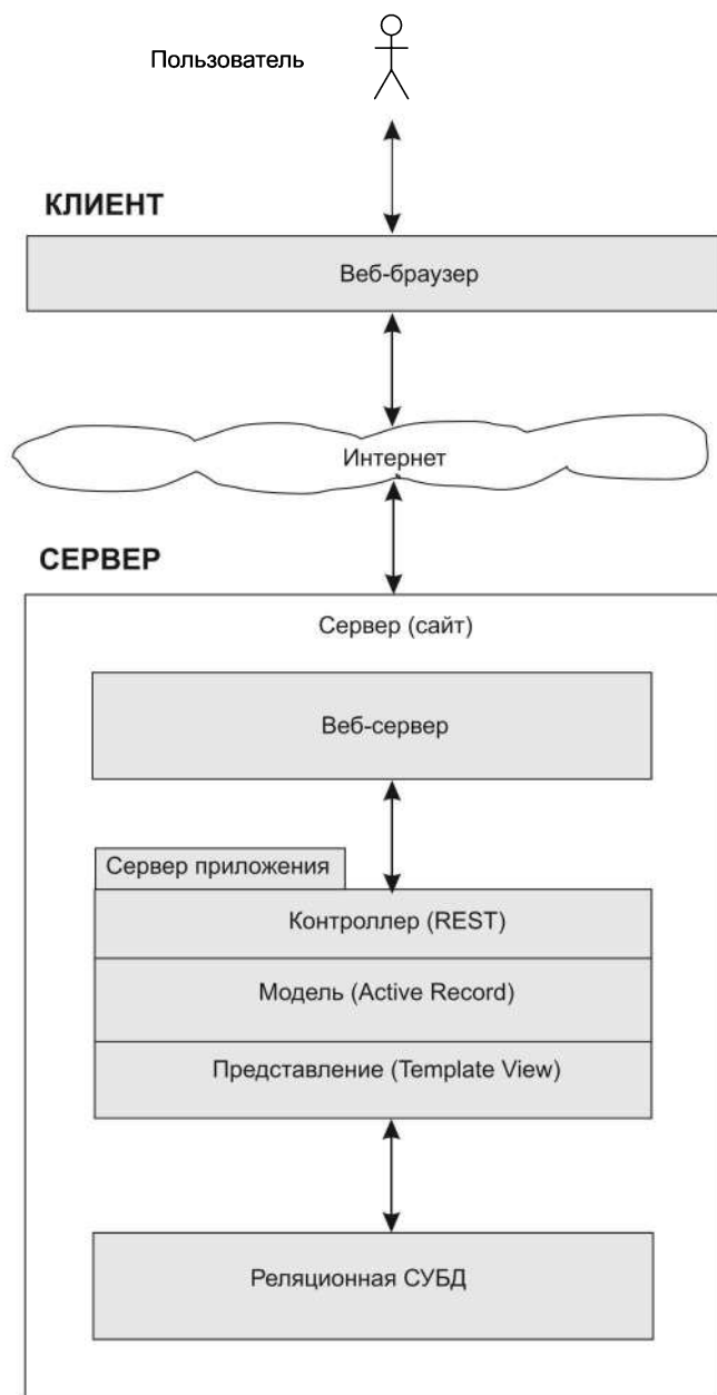
Рис. 19.5. Архитектура SaaS-приложения
