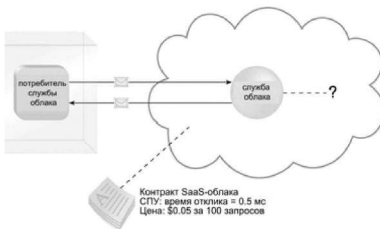
Рис. 19.3. Аренда SaaS-службы
