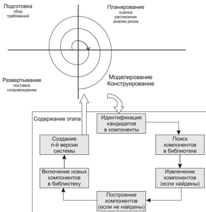
Рис. 1.6. Компонентно-ориентированная модель
