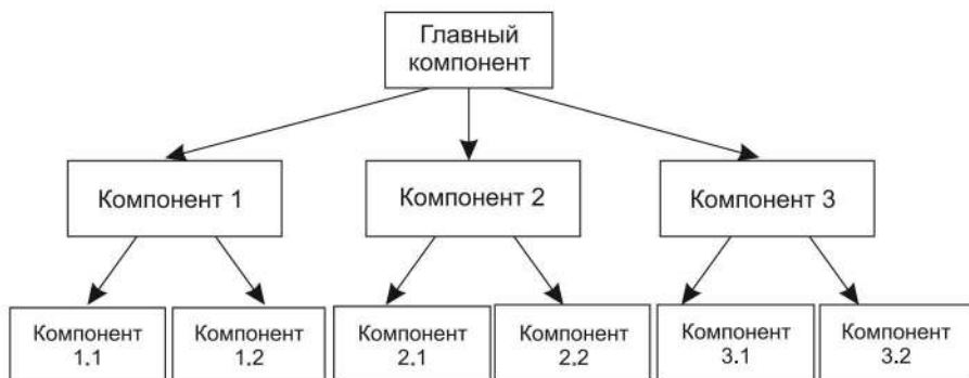
Рис. 6.11. Паттерн вызов-возврат
