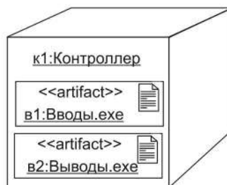
Рис. 10.77. Экземпляр узла
