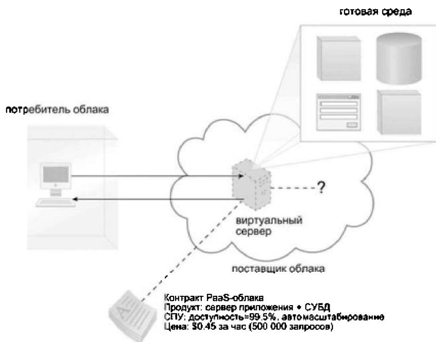
Рис. 19.2. Аренда PaaS-среды
