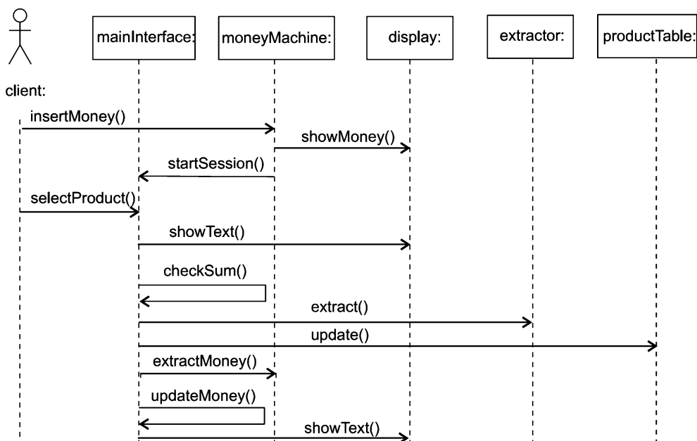
Рис. 13.28. Диаграмма последовательности для элемента Use Case ByCash
