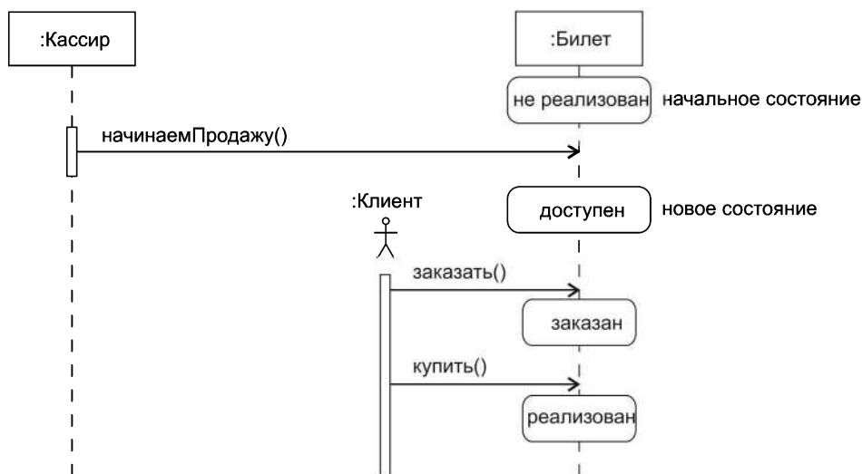
Рис. 9.32. Состояние объекта на диаграмме последовательности
