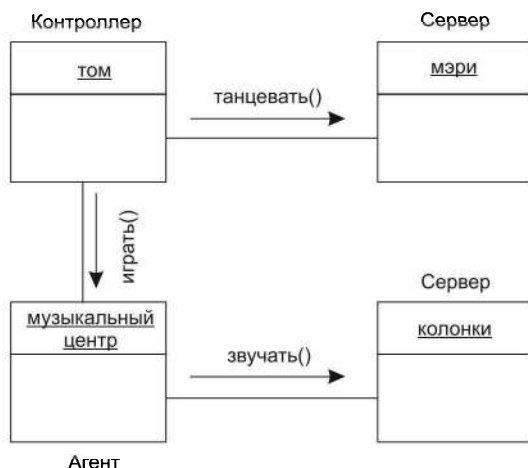
Рис. 8.5. Связи между объектами
