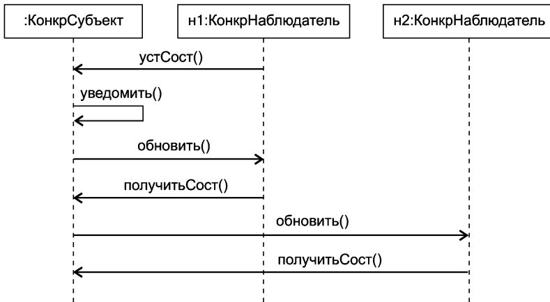
Рис. 10.48. Динамическая составляющая паттерна Наблюдатель
