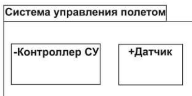
Рис. 10.2. Именованное пакета с отображением его содержания
