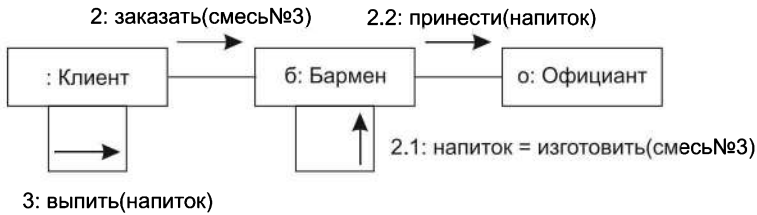
Рис. 9.23. Поток синхронных сообщений
