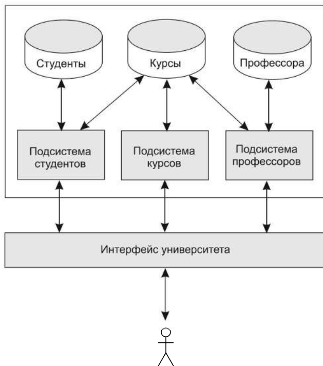
Рис. 18.1. Бункерная информационная система университета
