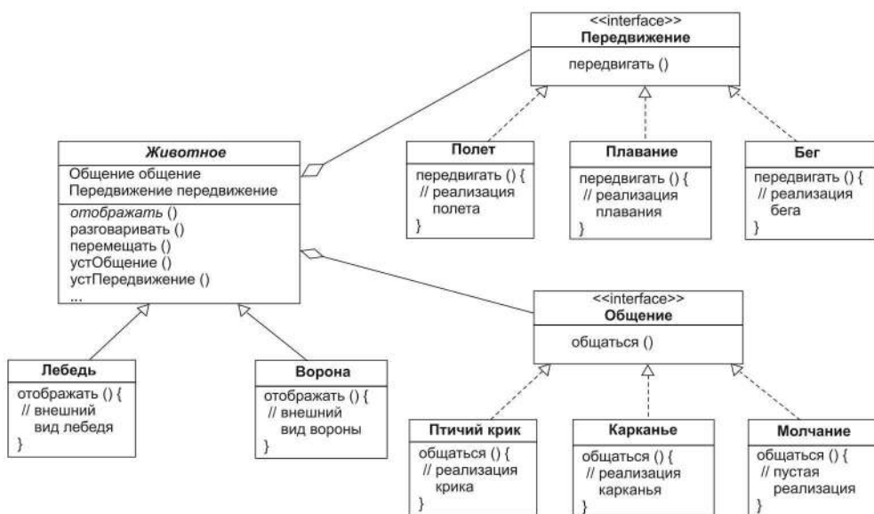
Рис. 10.41. Интерфейс и реализующие классы для операции общения
