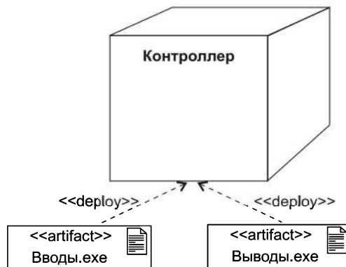
Рис. 10.76. Развертывание артефактов в узле
