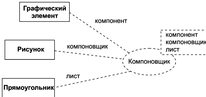
Рис. 10.53. Настройка паттерна Компоновщик
