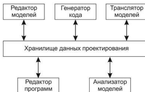
Рис. 6.5. Архитектура Case-системы на основе паттерна хранилища данных
