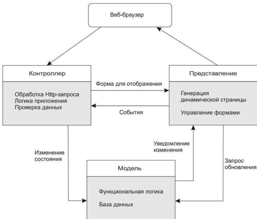
Рис. 6.4. Архитектура веб-системы на основе паттерна модель-представление-контроллер
