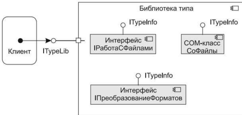
Рис. 10.71. Доступ к библиотеке типа
