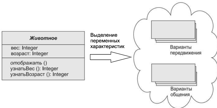
Рис. 10.38. Выделение переменных характеристик поведения
