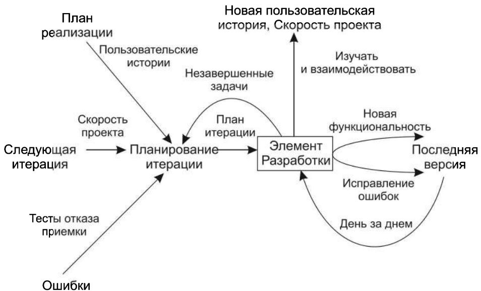
Рис. 13.32. Структура XP-итерации
