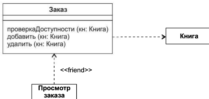
Рис. 10.27. Отношения зависимости
