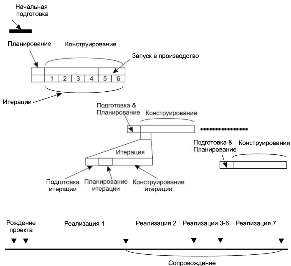
Рис. 1.7. Идеальный XP-процесс
