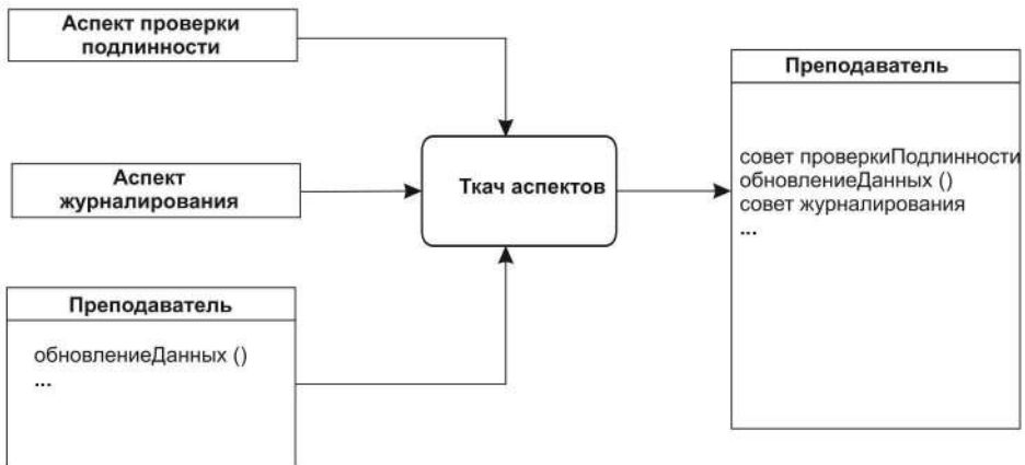
Рис. 10.60. Вплетение аспектов
