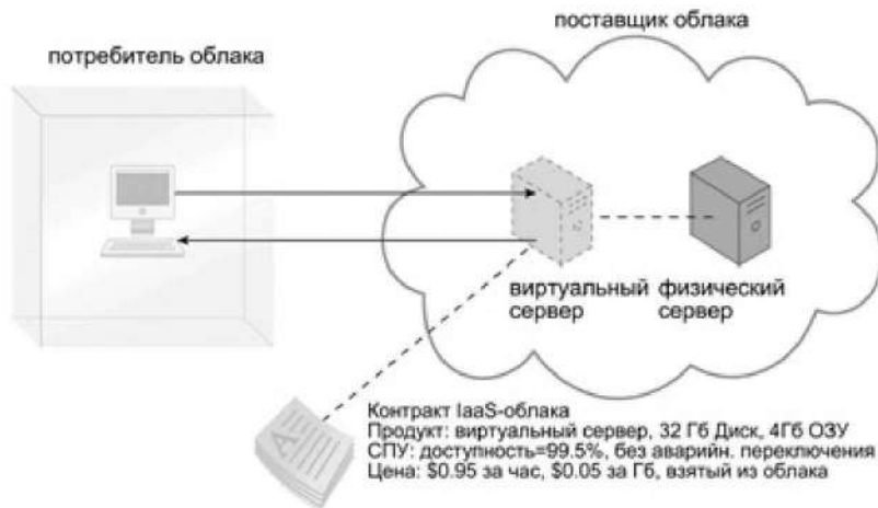
Рис. 19.1. Аренда IaaS-среды
