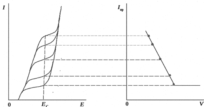
17-сурет. Зерттелетін қосылыстың активтілігіне сәйкес вольтамперметрлік I=f(E) және амперметрлік титрлеу I=f(V) қисықтары
