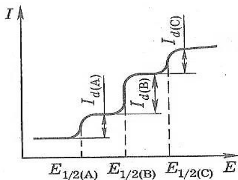
16-сурет. Құрамында тотықсызданатын бірнеше ион бар ерітіндінің полярограммалары
