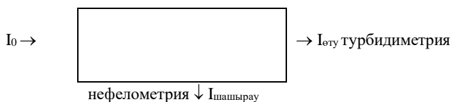
8-сурет. Нефелометриялық және турбидиметриялық өлшемі үшін жарық ағынының сызбанұсқасы
