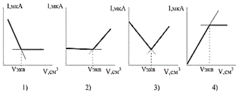
18-сурет. Амперметрлік титрлеу қисықтары 1) титрленетін зат активті; 2) титрант активті; 3) титрленетін зат және титрант активті; 4) реакция өнімі активті
