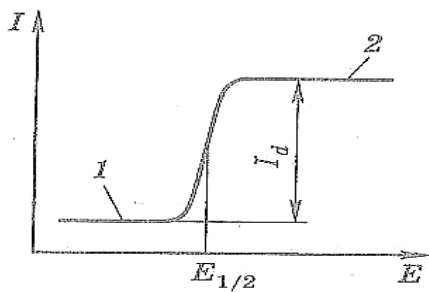
15-сурет. Волтамперметрлік тәуелділік
