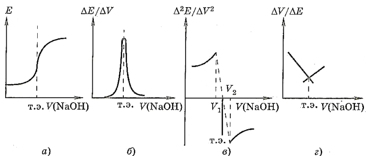
14-сурет. Потенциометрлік титрлеу қисықтары.
